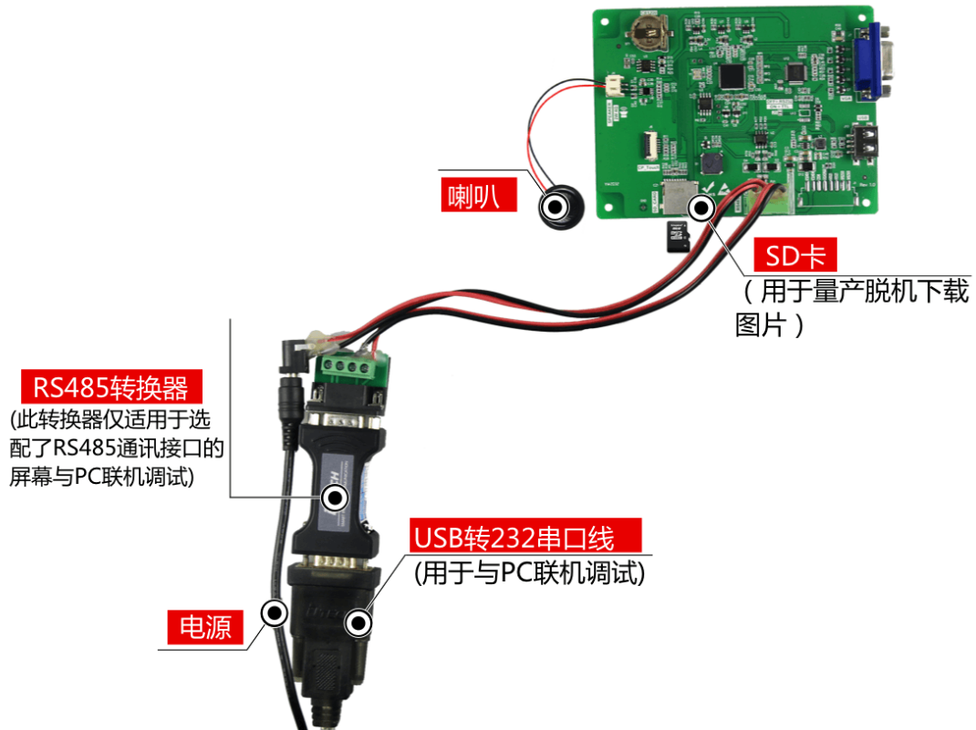
图 1-3 调试工具图
